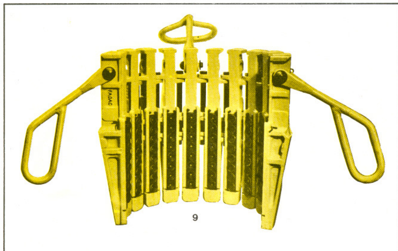
Lista de Repuestos para la Cuña CPV-L
