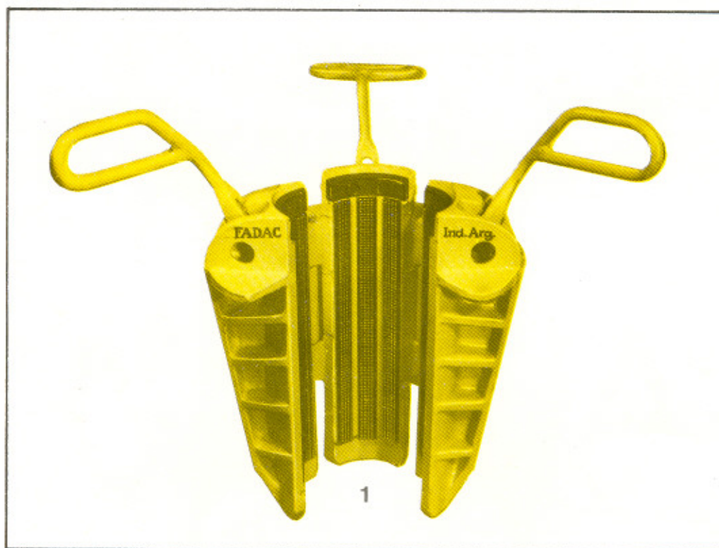
Lista de Repuestos para la Cuña CPV-E Extra larga
