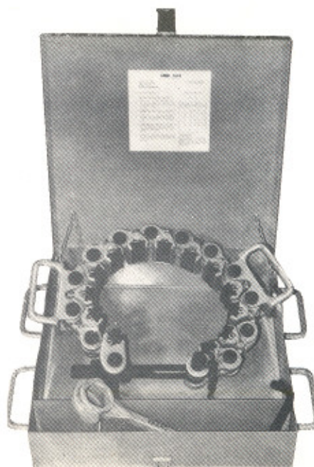
COLLARIN DE SEGURIDAD "CYJ" con llaves de ajuste y caja metálica
