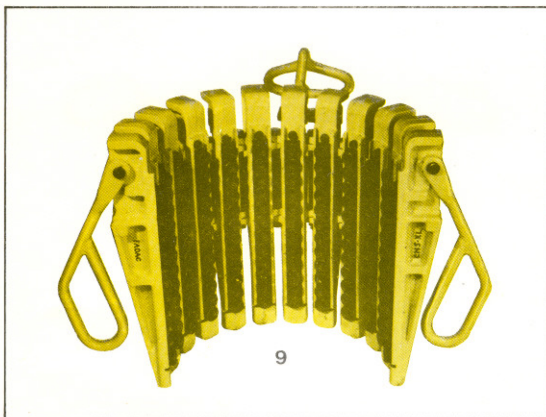
Lista de Repuestos para la Cuña CCV-E Extra larga
